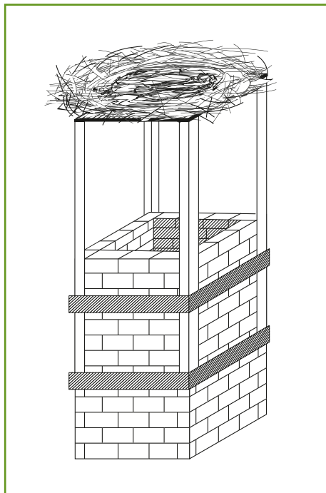
Schemat platformy na kominie
