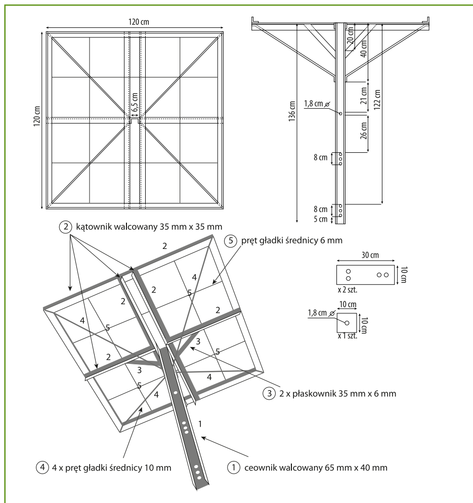
Platforma gniazdowa metalowa przeznaczona do montażu na słupach energetycznych
